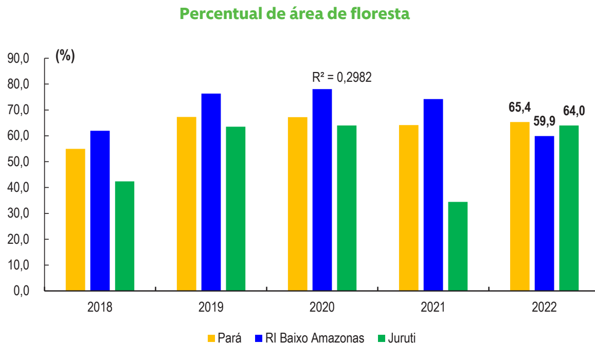
Gráfico 26: Percentual de área de floresta, Pará, Região de Integração do Baixo Amazonas e Juruti, 2018 a 2022.
