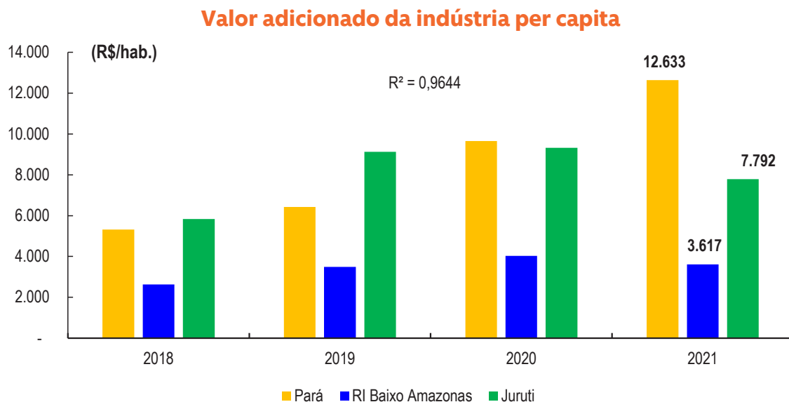
Gráfico 17: Valor adicionado da indústria per capita, Pará, Região de Integração do Baixo Amazonas e Juruti, 2018 a 2021.
